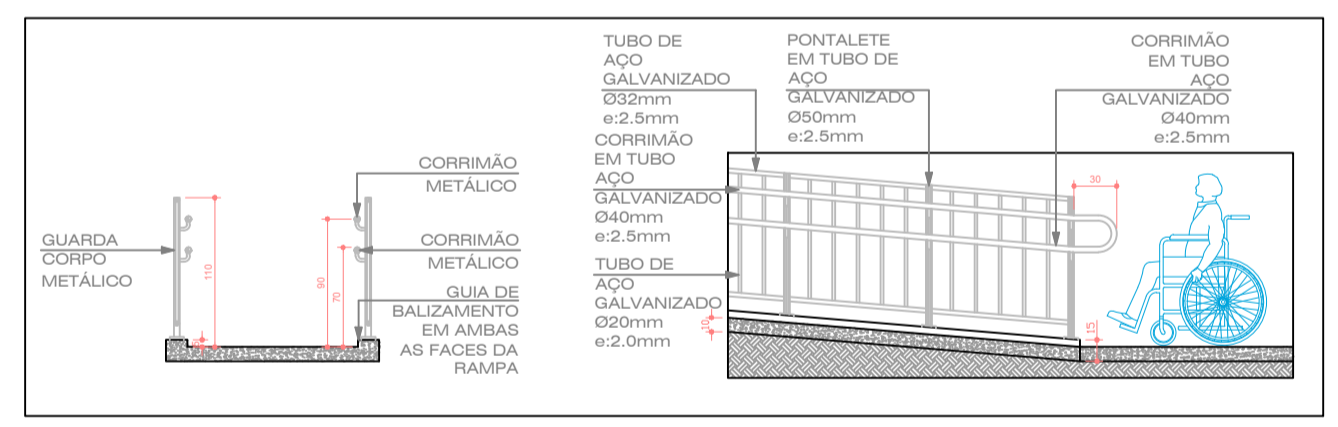
Detalhes Guarda-Corpo Rampas Acessíveis Escala: 1:50
