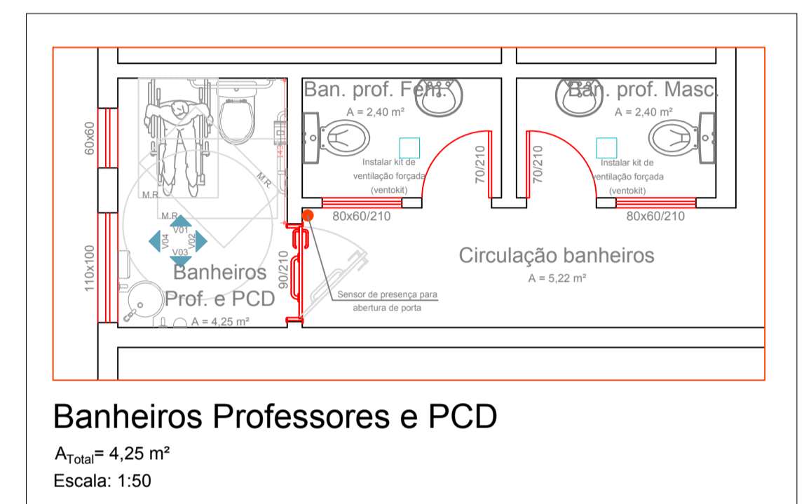
Detalhes Banheiros Acessíveis Térreo
