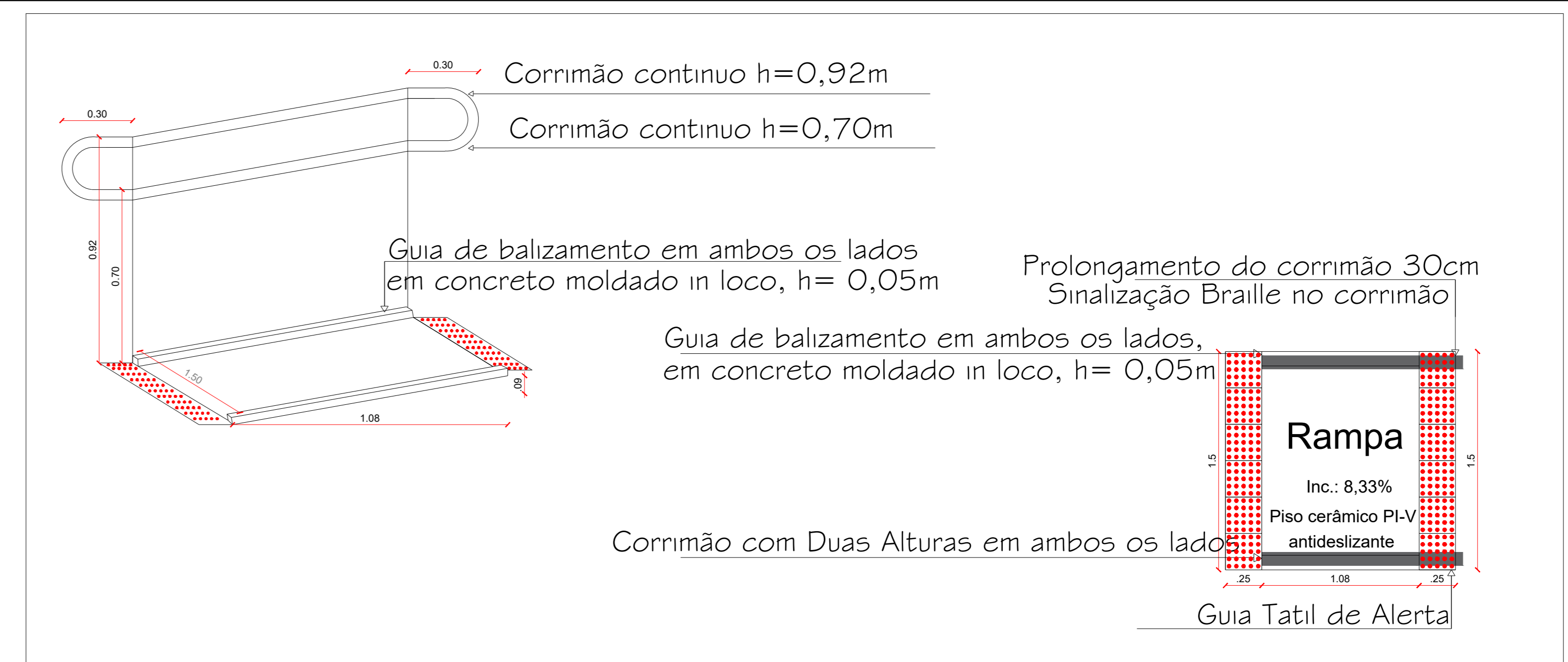
DETALHE 04 – Rampa acesso banheiro PCD da Câmara de Vereadores Esc: 1:25
