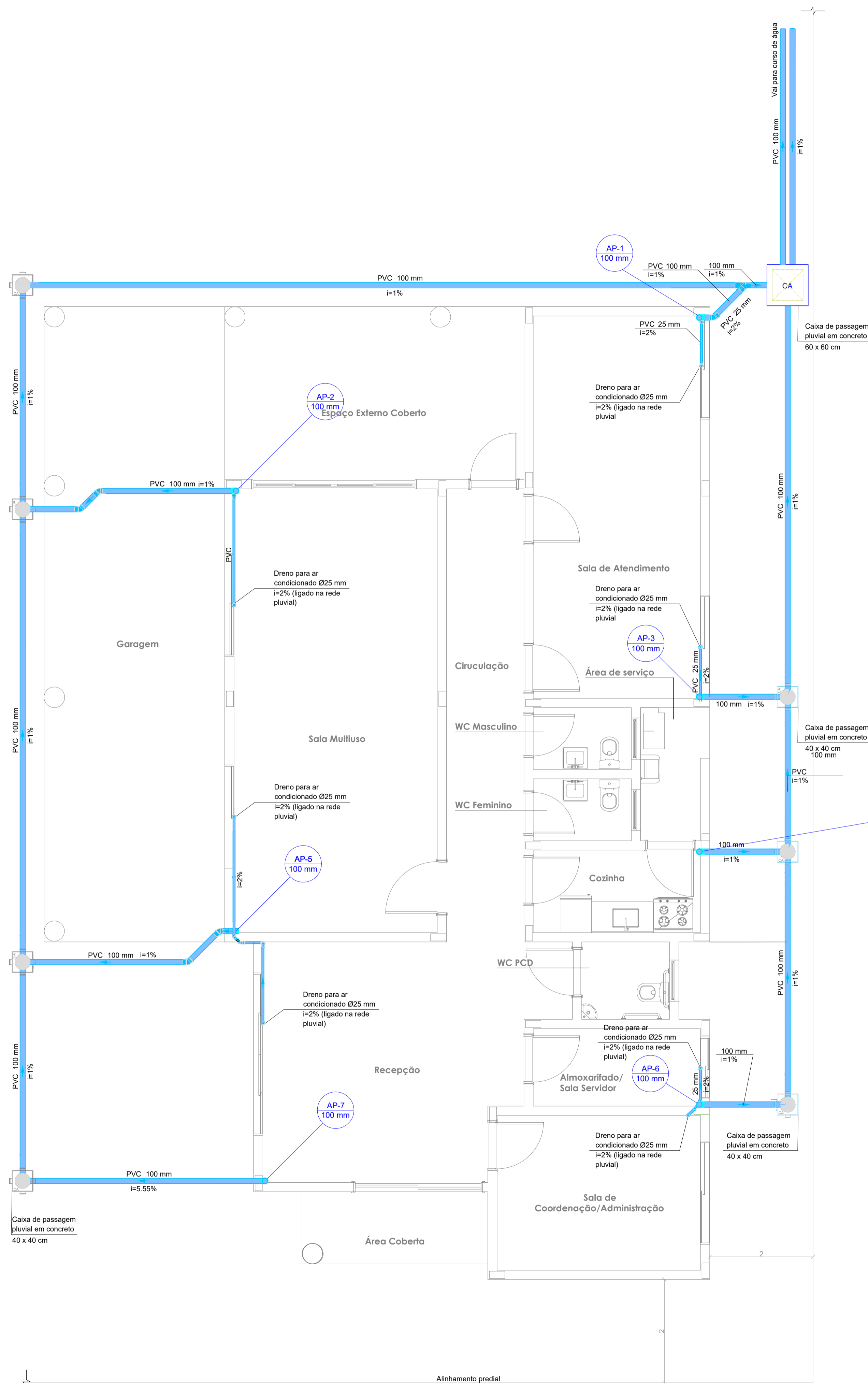
Planta Baixa Pluvial Escala 1:50
