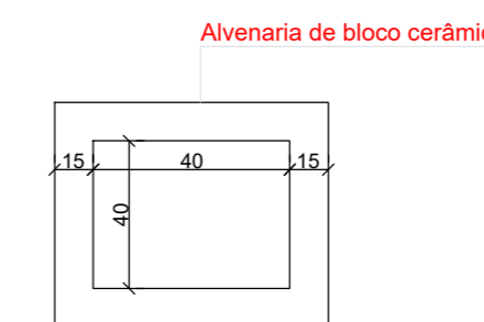
Caixa de passagem Lógica e Telefone Planta baixa - ESC. 1:25
