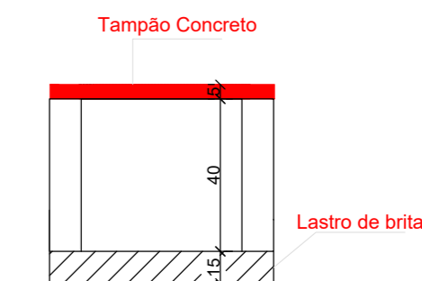
Caixa de passagem Lógica e Telefone Corte - ESC. 1:25
