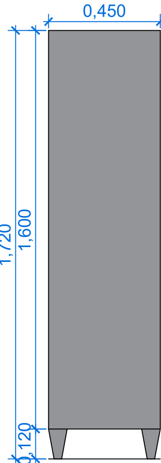
VISTA LATERAL
