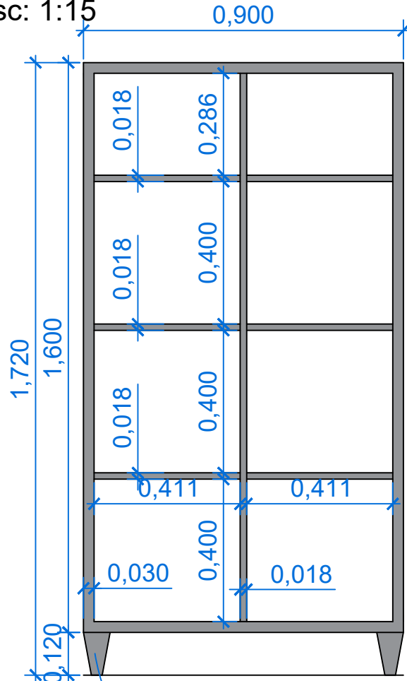
VISTA INTERNA
