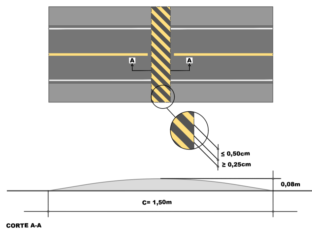
CORTE A-A
